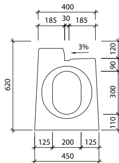
Widok "a" I-2-V0 - wpust
