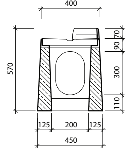
I-2-V0 - prawy - skrzynka odpływowa z krawężnikiem 7 cm z żeliwną ramą i pokrywą pełną z tworzywa dla klasy D400
