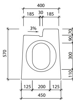
Widok "b" I-2-V0 - wpust
