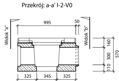
I-2-V0 - prawy - skrzynka odpływowa z krawężnikiem 7 cm z żeliwną ramą i pokrywą pełną z tworzywa dla klasy D400
