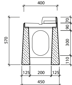
Przekrój: b-b' I-2-V0
