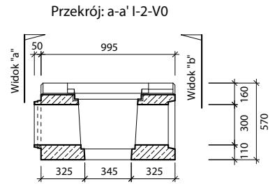
I-2-V0 - lewy - skrzynka odpływowa z krawężnikiem 7 cm z żeliwną ramą i pokrywą pełną z tworzywa dla klasy D400
