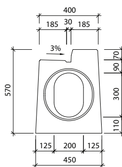
Widok "b" I-2-V0 - pióro
