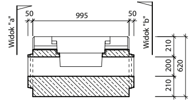
Przekrój: a-a' I-3-CS
