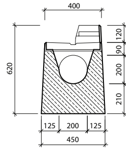
Przekrój: b-b' I-3-CS
