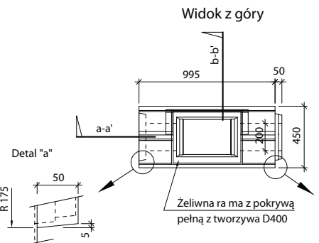
Widok "a" I-3-V0 - wpust
