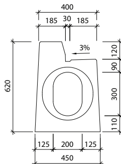
Widok "a" I-3-VU - wpust/wpust
