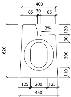
Widok "a" I-3-V0 - wpust
