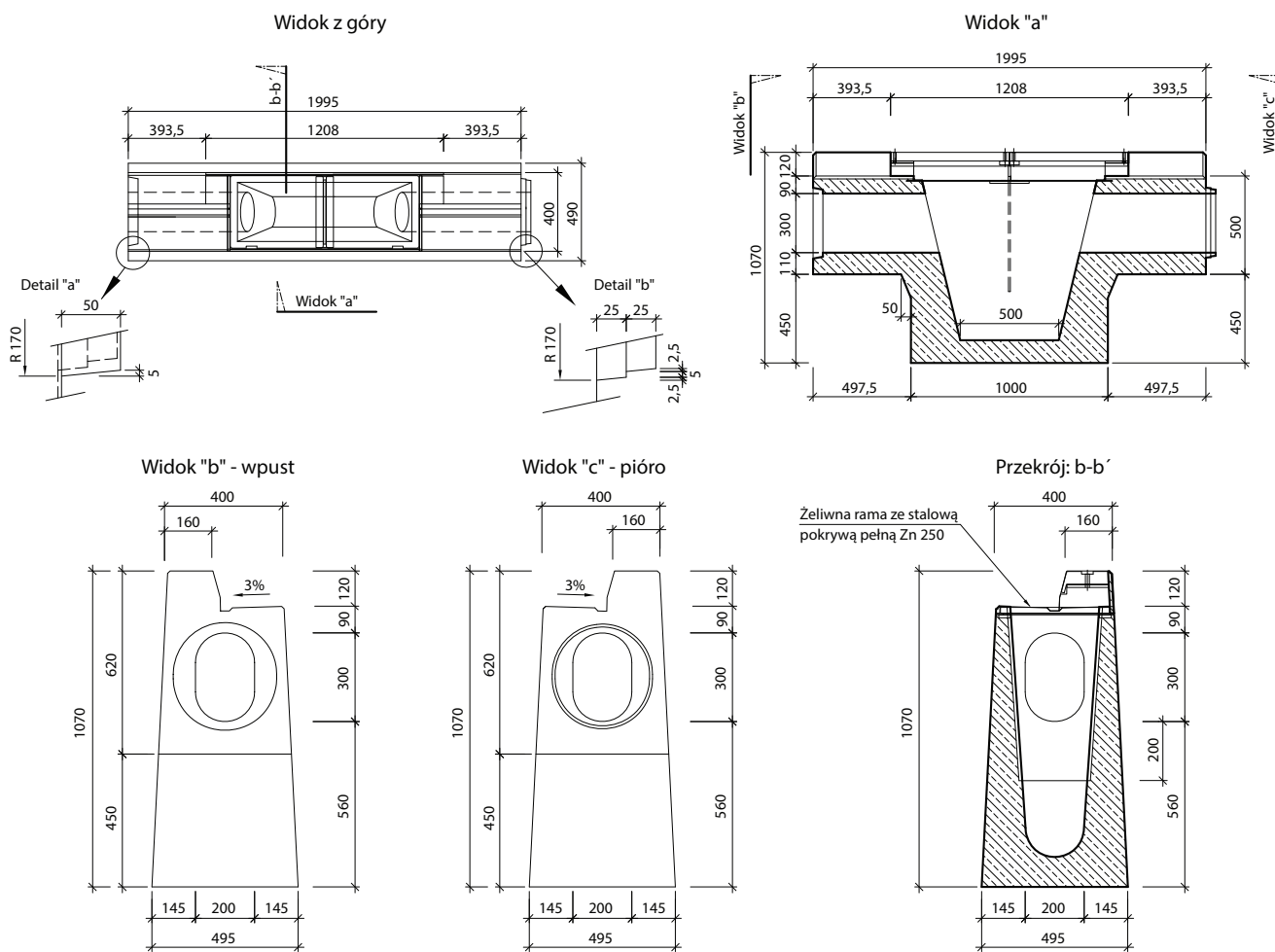
I-3-PP - prawy - przegroda przeciwpożarowa z krawężnikiem 12 cm z żeliwną ramą i stalową pokrywą pełną
