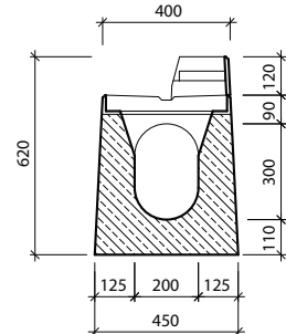
Przekrój: b-b' I-3-C0
