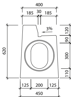
Widok "a" I-3-C0 - pióro
