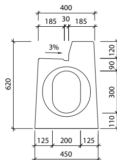
Widok "b" I-3-C0 - wpust
