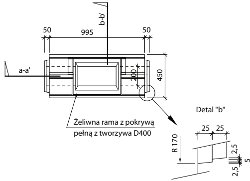
Widok "a" I-3-CS - pióro/pióro
