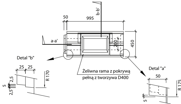
Widok "a" I-3-C0 - pióro
