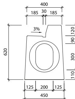
Widok "b" I-3-VU - wpust/wpust
