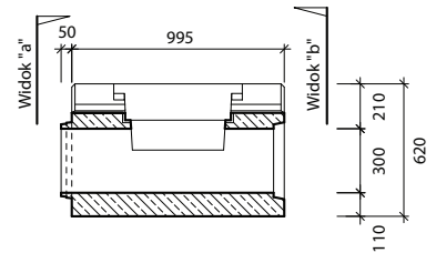
Przekrój: a-a' I-3-C0
