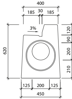
Widok "b" I-3-CS - pióro/pióro
