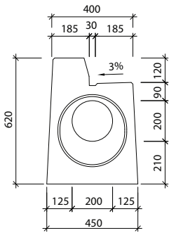
Widok "a" I-3-CS - pióro/pióro
