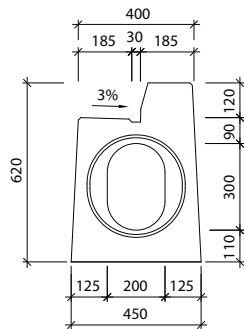
Widok "b" I-3-V0 - pióro
