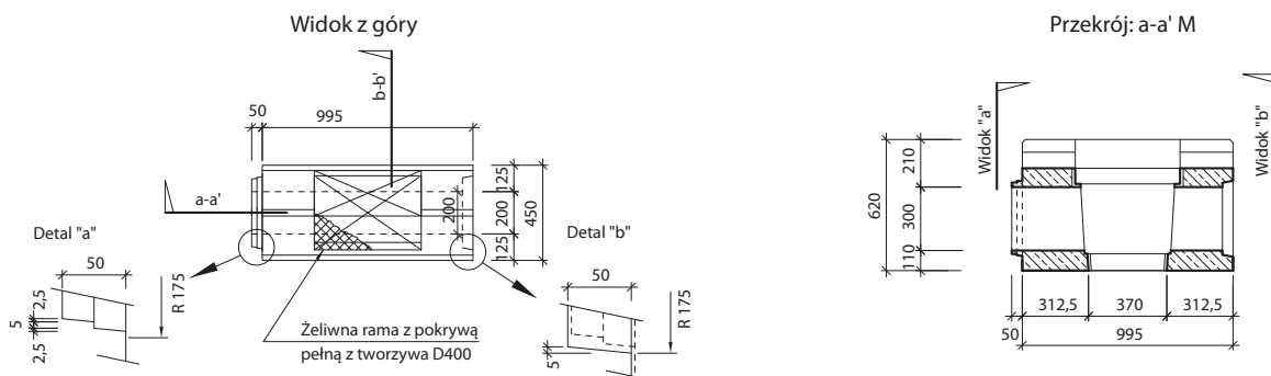
I-5-V0 - lewy - skrzynka odpływowa z krawężnikiem 12 cm z żeliwną ramą i pokrywą pełną z tworzywa dla klasy D400
