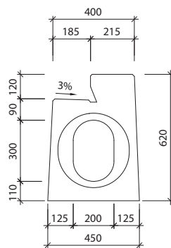
Widok "b" I-5-V0 - wpust
