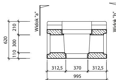
Przekrój: a-a' I-5-VU
