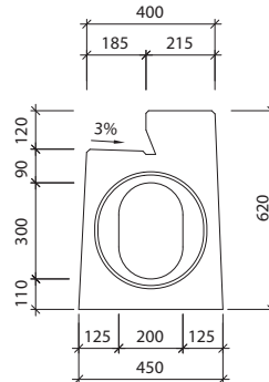
Widok "b" I-5-V0 - pióro
