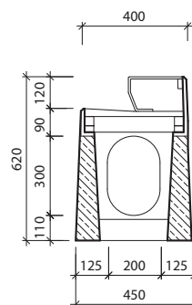
Przekrój: b-b' I-5-V0
