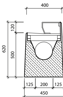
Przekrój: b-b' I-5-CS
