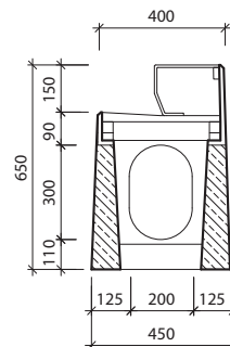
I-6-V0 - prawy - skrzynka odpływowa z krawężnikiem 15 cm z żeliwną ramą i pokrywą pełną z tworzywa dla klasy D400
