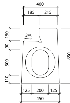
Widok "b" I-6-C0 - wpust
