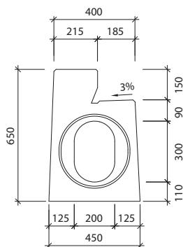
Widok "a" I-6-V0 - pióro
