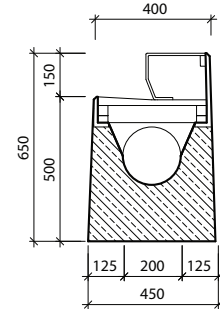
Przekrój: b-b' I-6-CS
