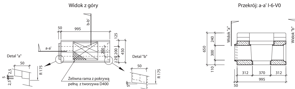
Przekrój: a-a' I-6-V0
