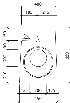
Widok "b" I-6-CS - pióro/pióro
