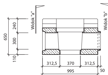
Przekrój: b-b' I-6-V0
