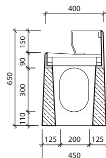
Przekrój: b-b' I-6-V0
