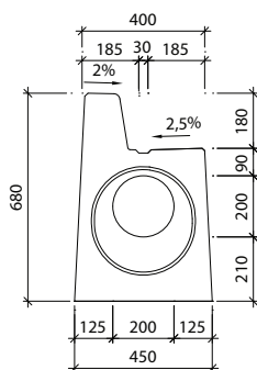
I-7-C0 - lewy - element rewizyjny z krawężnikiem 18 cm z ramą żeliwną i pokrywą stalową dla klasy D400
