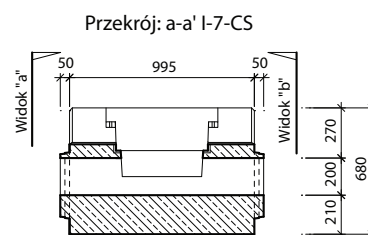
I-7-CS - element rewizyjny pióro/pióro z krawężnikiem 18 cm z ramą żeliwną i pokrywą stalową dla klasy D400
