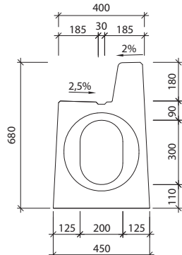
Widok "b" I-7-VU - wpust/wpust
