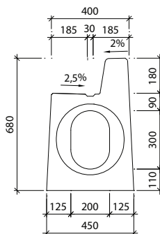
Widok "b" I-7-V0 - wpust
