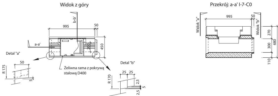
Widok "a" I-7-C0 - wpust
