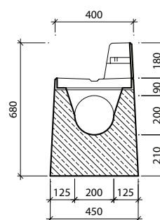
I-7-C0 - lewy - element rewizyjny z krawężnikiem 18 cm z ramą żeliwną i pokrywą stalową dla klasy D400
