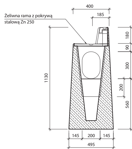
Przekrój: b-b' I-7-PP
