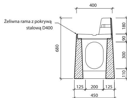
Przekrój: b-b' I-7-VU
