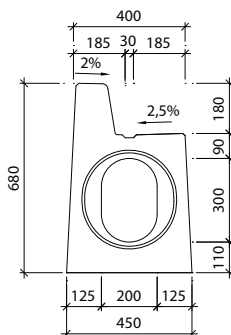
Widok "a" I-7-V0 - pióro
