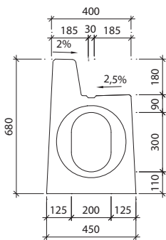
Widok "a" I-7-C0 - wpust
