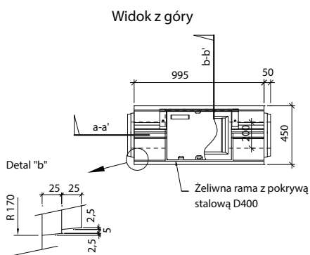
I-7-CS - element rewizyjny pióro/pióro z krawężnikiem 18 cm z ramą żeliwną i pokrywą stalową dla klasy D400
