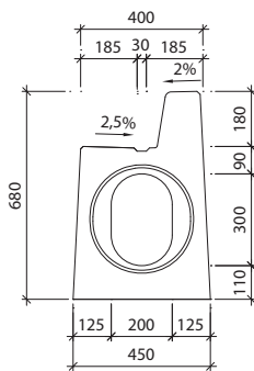
Widok "b" I-7-C0 - pióro
