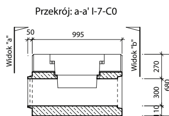
I-7-C0 - lewy - element rewizyjny z krawężnikiem 18 cm z ramą żeliwną i pokrywą stalową dla klasy D400
