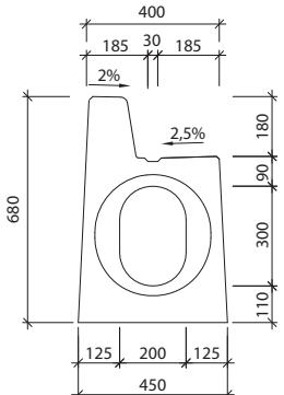
Widok "a" I-7-VU - wpust/wpust
