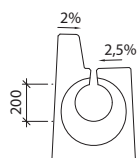
Widok "b" - wpust
