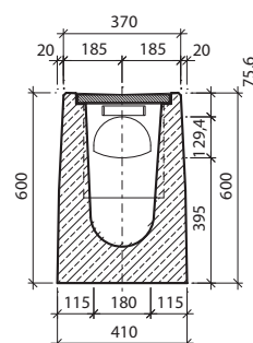
Przekrój: b-b' T-1-PP
