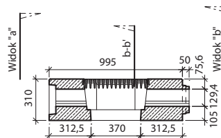
Przekrój: a-a' T-1-V0
