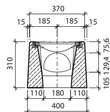
Przekrój: b-b' T-1-VU
