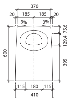
Widok "a" T-1-PP - wpust
