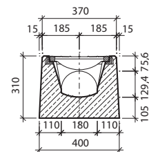
Przekrój: b-b' T-1-C0
